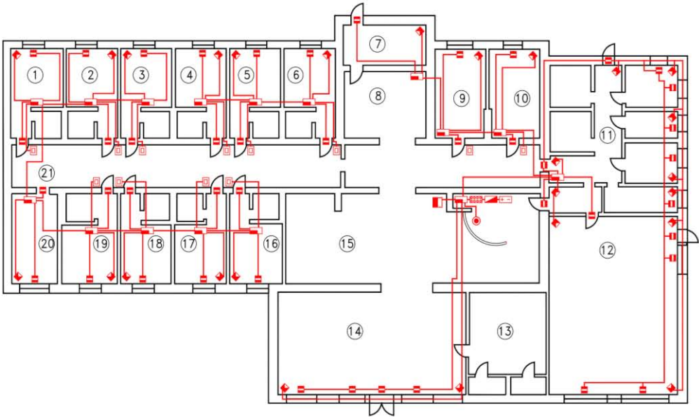
Рекомендуемый план расположения извещателей СОС в помещениях
